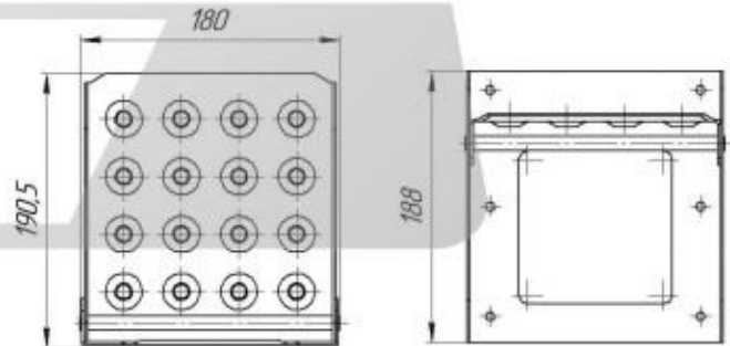
Подножка в сложенном виде
