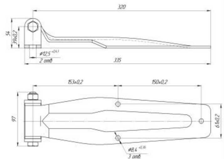
F06 Hinge (Zn, SS) – 6306034-13
